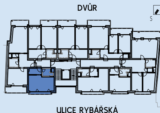
PŮDORYS 3.NP
